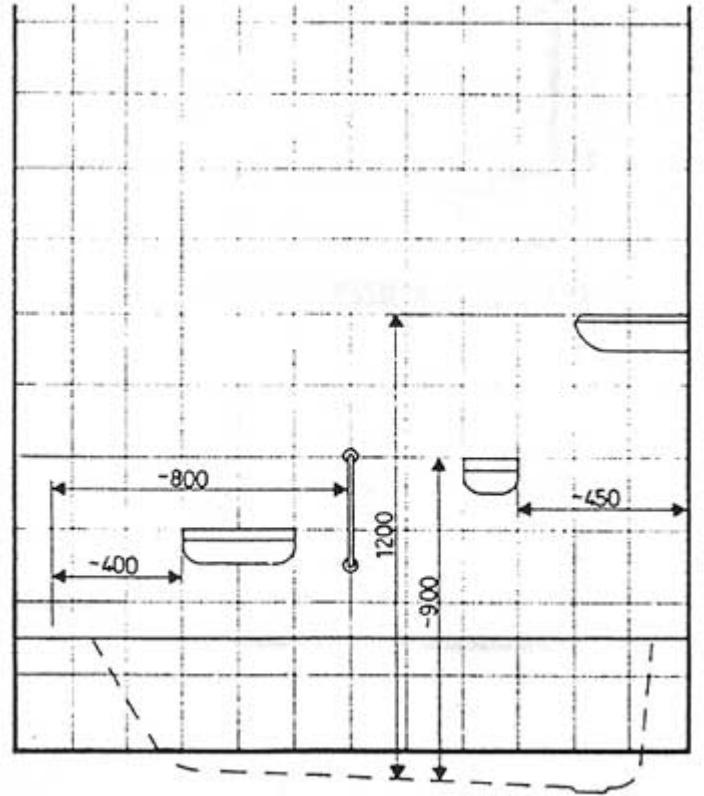
Küvet aksesuarlarının yer ve ölçüleri
