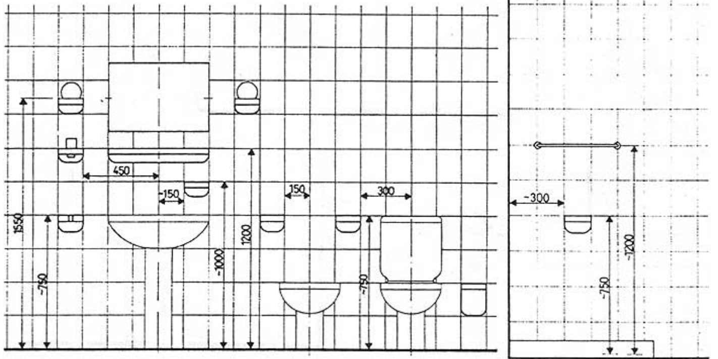
Seramik aksesuarların kullanıldığı yer ve ölçüleri
