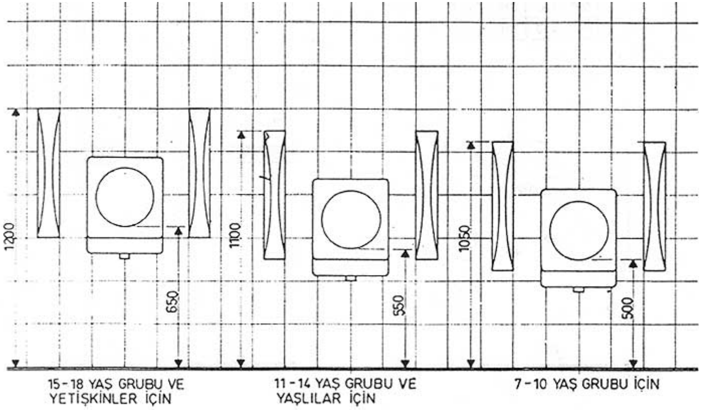
pisvarların yaş gruplarına göre yüksekliği
